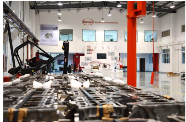
独自のデザイン／高速プロセスの機能を備え、 年間 40 万個以上のエンジンブロックをシーリング可能
